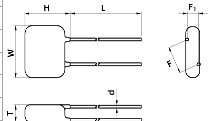
直型引线 Straight Lead
