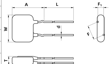
外弯型引线 Outward Crimp
