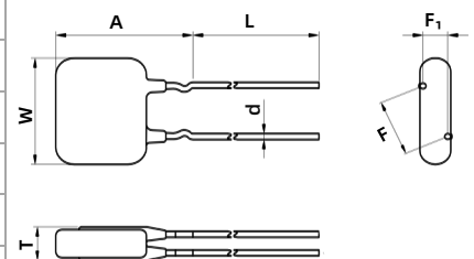
内弯型引线 Inward Crimp
