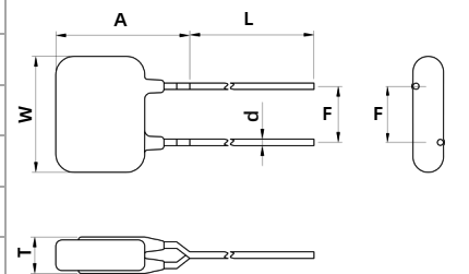
Y 型引线 Inline Crimp
